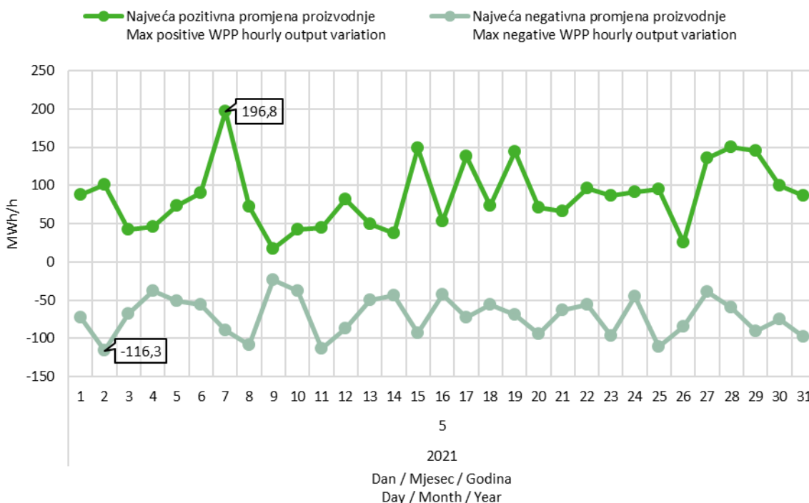
Slika 9 Maksimalna pozitivna i maksimalna negativna promjena satne proizvodnje VE u svibnju 2021. godine
