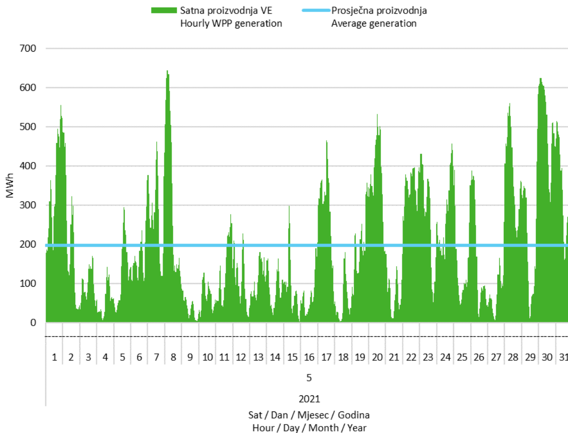
Slika 2 Satna proizvodnja svih vjetroelektrana u svibnju 2021. godine
