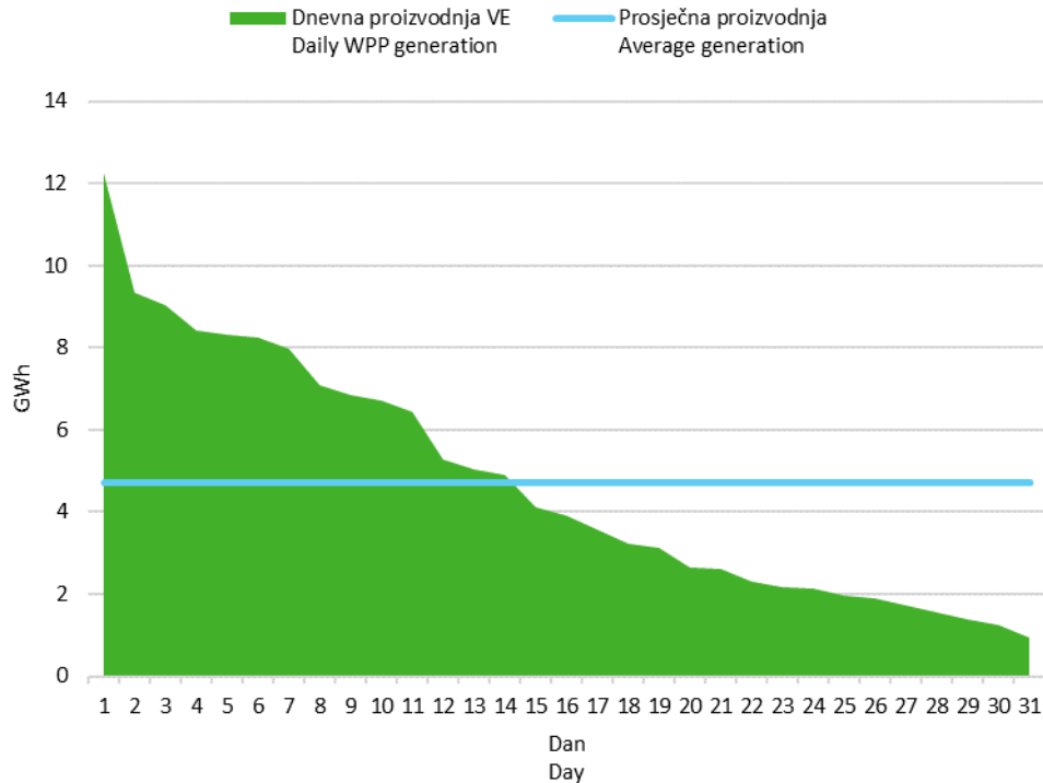
Slika 6 Krivulja trajanja dnevne proizvodnje vjetroelektrana u svibnju 2021. godine
