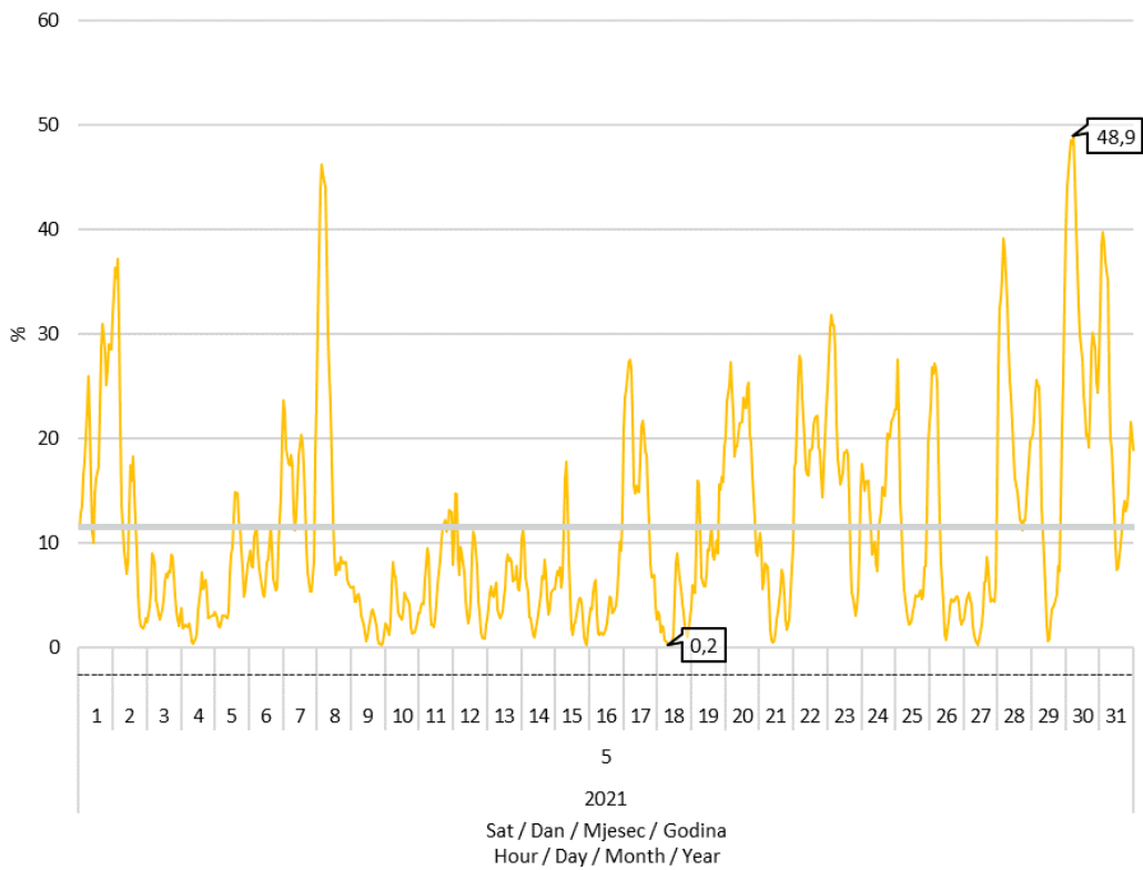
Slika 8 Udio proizvodnje vjetroelektrana u pokrivanju satnog opterećenja elektroenergetskog sustava u svibnju 2021. godine
