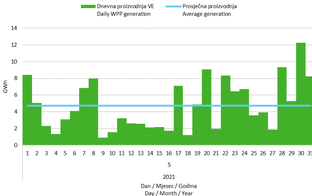
Slika 5 Dnevna proizvodnja svih vjetroelektrana u svibnju 2021. godine Figure 5 Daily generation of all wind power plants in May 2021
