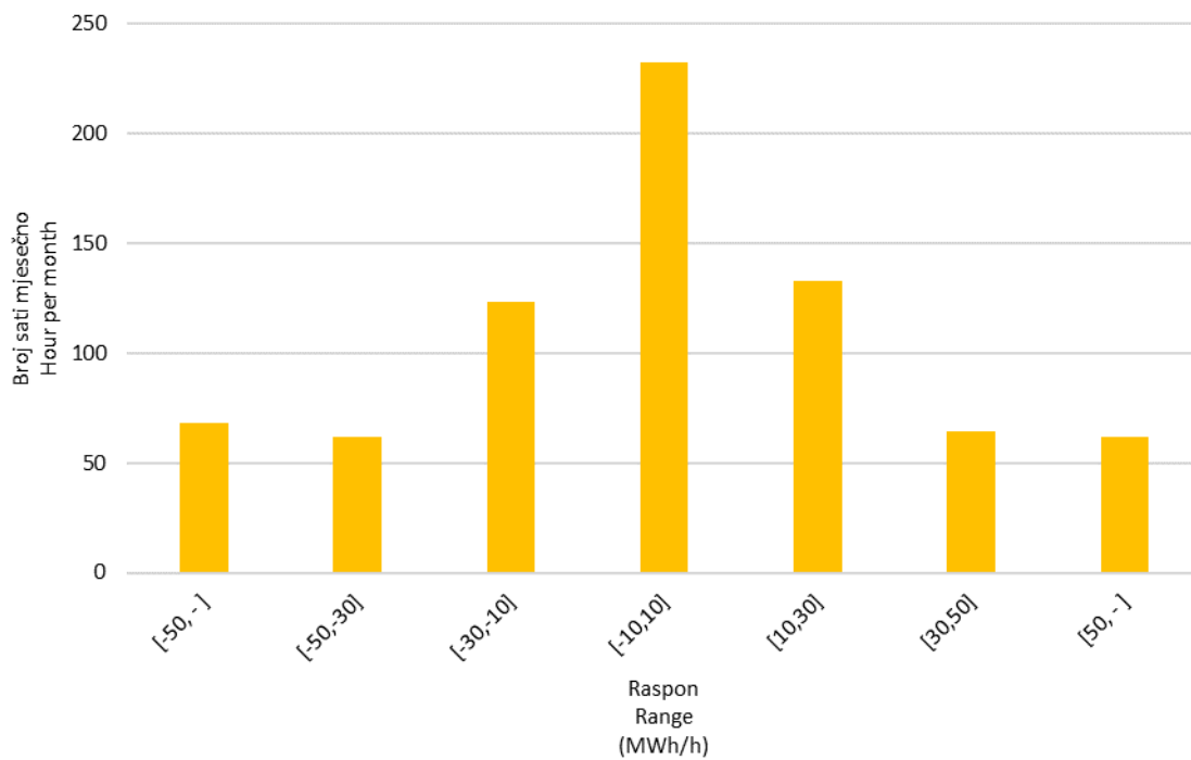
Slika 10 Statistička raspodjela satnih promjena proizvodnje VE u svibnju 2021. godine
