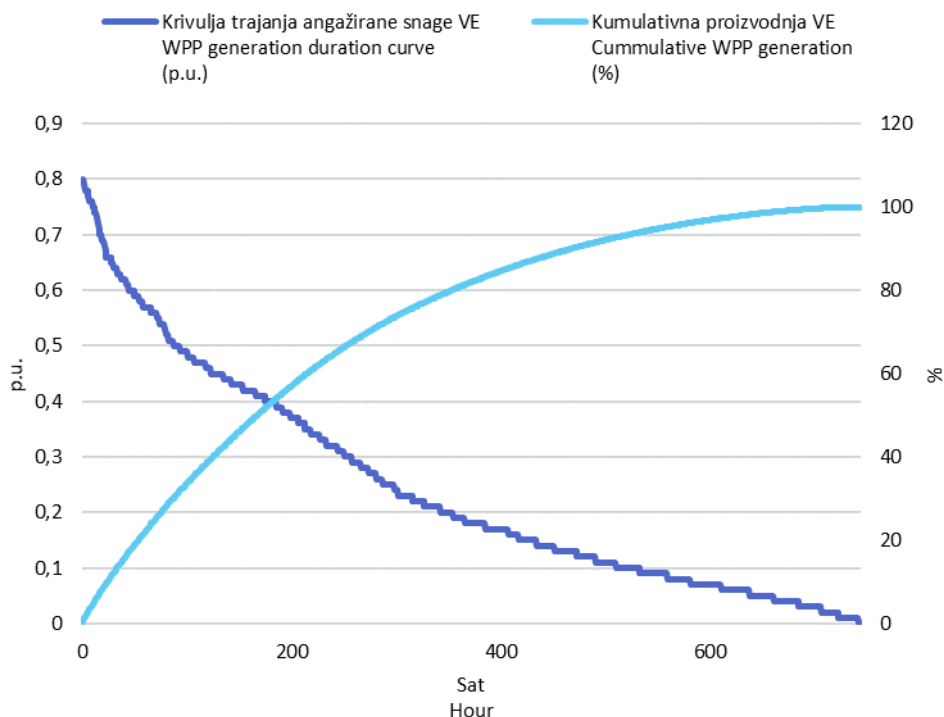
Slika 3 Krivulja trajanja angažirane snage svih VE i kumulativna proizvodnja VE u svibnju 2021. godine u jediničnim vrijednostima
