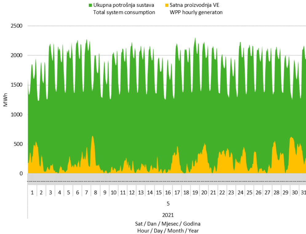
Slika 7 Usporedba satnog dijagrama opterećenja sustava i proizvodnje vjetroelektrana u svibnju 2021. godine
